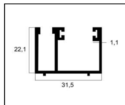
VT-010 TRILHO INFERIOR PESO: 0,300 Kg/m
