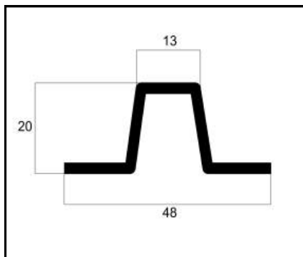
DS-192 PERFIL TRAPÉZIO PESO: 0,382 Kg/m
