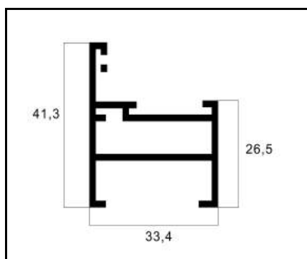
ASU-279 MARCO LATERAL DA PORTA PESO: 0,639 Kg/m
