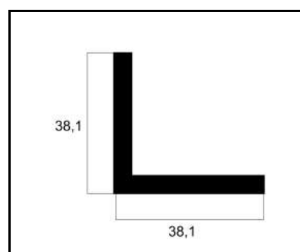
CT-08 CANTONEIRA 1 1/2" X 1/8 PESO: 0,723 Kg/m
