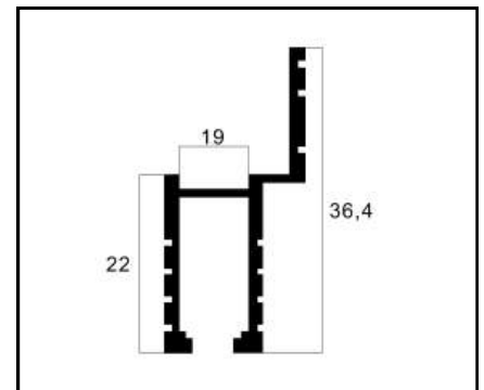
BXS-07 CADEIRINHA PESO: 0,189 Kg/m
