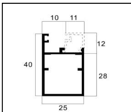
25-216 PESO: 0,495 Kg/m
