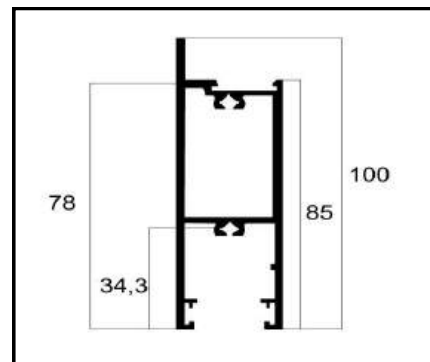
ALG-07 TRAVESSA PESO: 1,315 Kg/m
