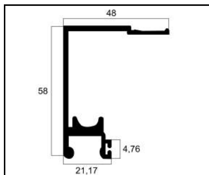
VT10-01 TRILHO SUPERIOR PESO: 0,726 Kg/m
