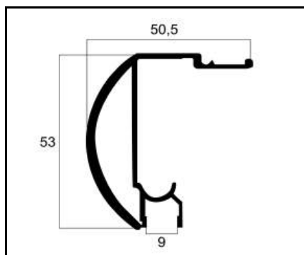
VT-201 TRILHO SUPERIOR PESO: 0,520 Kg/m
