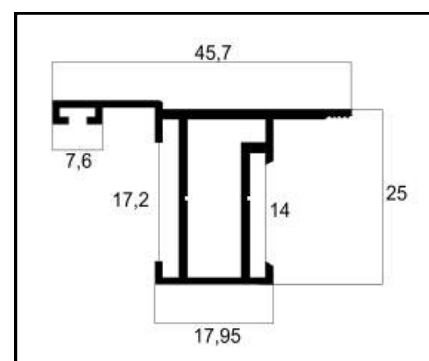
ASU-200 PESO: 0,382 Kg/m
