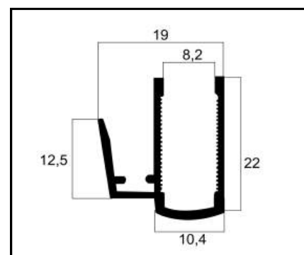
VT-252 MÃO AMIGA PESO: 0,199 Kg/m
