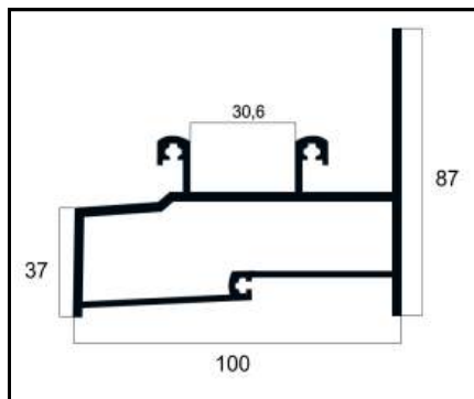
ALG-05 TRILHO INTERMEDIÁRIO INFERIOR PESO: 1,999 Kg/m
