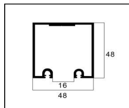
VT10-09 TRILHO SUPERIOR PESO: 0,839 Kg/m
