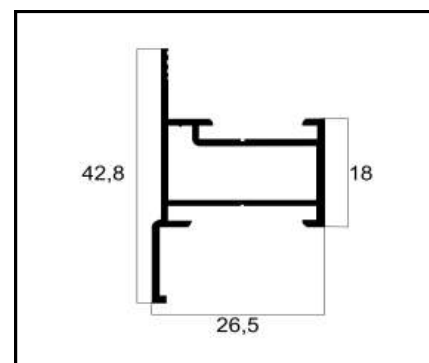
ASU-081 FOLHA LATERAL E INFERIOR PESO: 0,356 Kg/m
