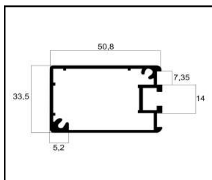
ACG-077 COLUNA PESO: 0,710 Kg/m
