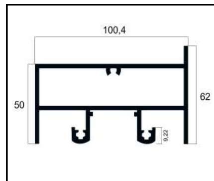
ALG-04 TRILHO INTERMEDIÁRIO SUPERIOR PESO: 1,789 Kg/m
