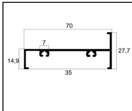
AMT-02 PEITORIL 70 PESO: 0,465 Kg/m
