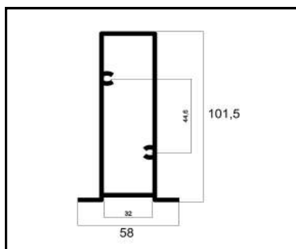
ALG-176 PERFIL COLUNA PESO: 1,437 Kg/m
