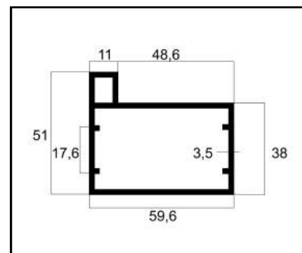
AMT-03 MONTANTE 60 PESO: 0,607 Kg/m
