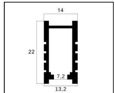
BXS-03 MONTANTE PESO: 0,176 Kg/m
