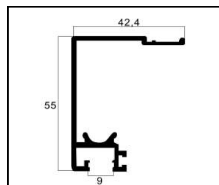
VT-01 TRILHO SUPERIOR PESO: 0,553 Kg/m
