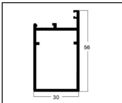
30-08 PESO: 0,721 Kg/m
