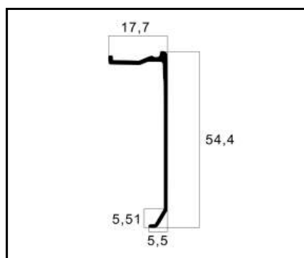
VT-087 CAPA PESO: 0,199 Kg/m
