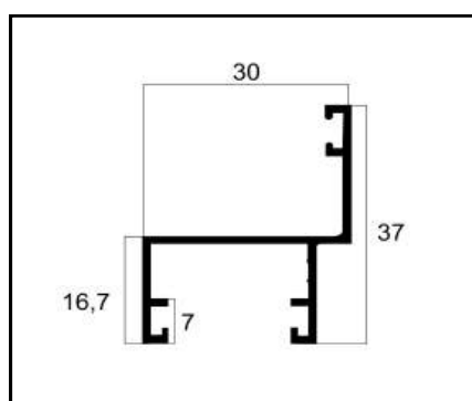
25-02 MARCO P/ MAXIAM AR PESO: 0,345 Kg/m
