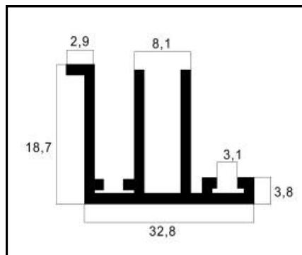
ALH-02 PERFIL MÃO AMIGA DESLIZANTE (TRILHO) PESO: 0,312 Kg/m
