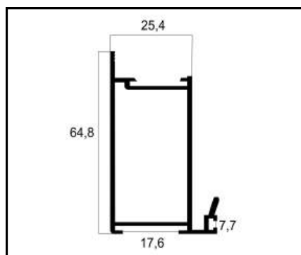
ASU-242 FOLHA MÃO AMIGO EXTERNO PESO: 0,720 Kg/m
