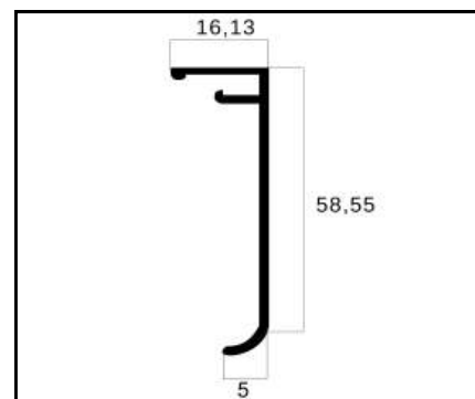
BXT-03 CAPA PESO: 0,180 Kg/m
