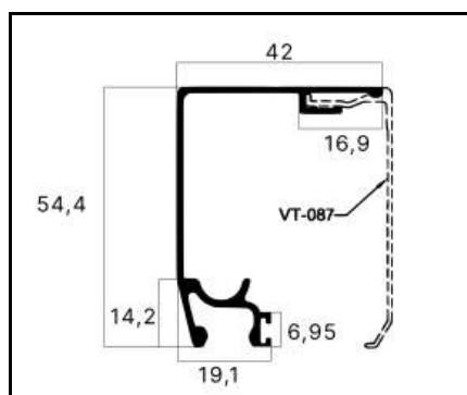
VT-086 TRILHO SUPERIOR PESO: 0,472 Kg/m
