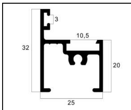
25-312 PESO: 0,393 Kg/m
