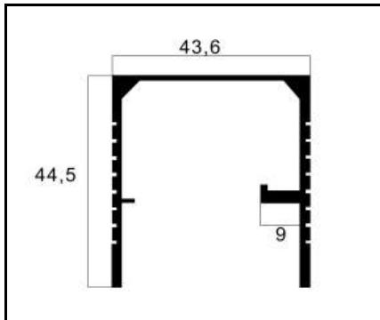
BXS-01 CHAPÉU QUADRADO PESO: 0,513 Kg/m
