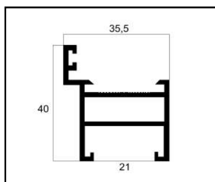
30-023 BATENTE DA PORTA PESO: 0,702 Kg/m
