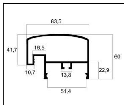
ACG-083 SUPERIOR PESO: 1,231 Kg/m
