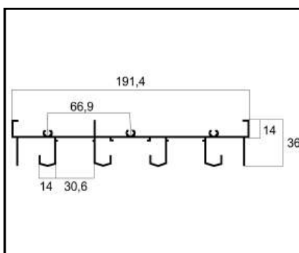
ALG-070 MARCO SUPERIOR 4 FOLHAS PESO: 1,867 Kg/m
