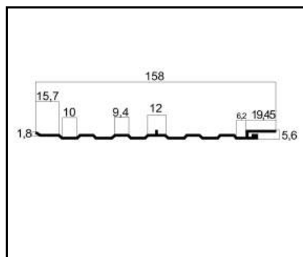
ALB-03 PESO: 0,713 Kg/m
