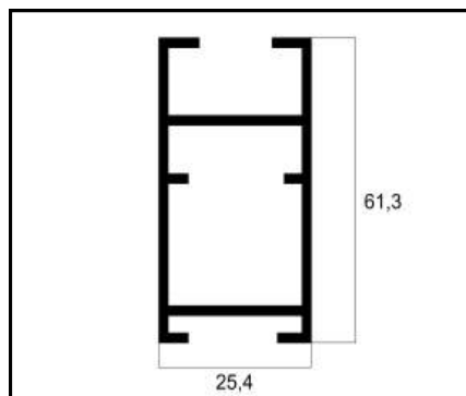
ASU-241 MONTANTE DA FOLHA PESO: 0,807 Kg/m
