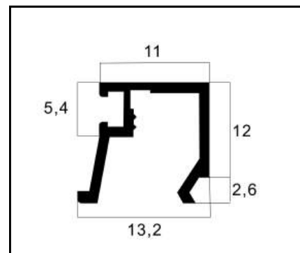
25-201 BAGUETE PESO: 0,114 Kg/m
