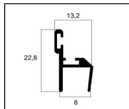
VT-099 CADEIRINHA / BATENTE CENTRAL PESO: 0,171 Kg/m
