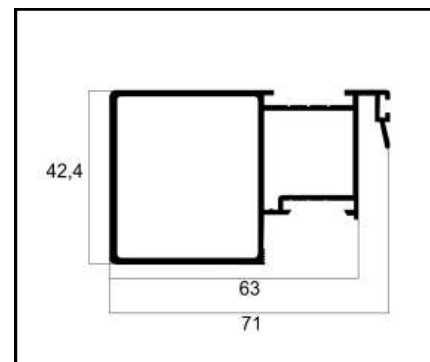
ASU-049 MÃO AMIGO EXTERNO C/ REFORÇO PESO: 1,011 Kg/m
