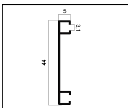
MV-092 TRILHO INFERIOR PESO: 0,129 Kg/m
