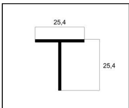
ALB-08 PERFIL "T" 1 X 1,2 MM PESO: 0,186 Kg/m
