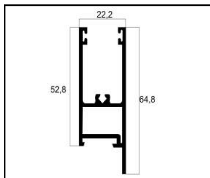
ASU-246 FOLHA INFERIOR HORIZONTAL PESO: 0,707 Kg/m
