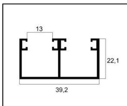
VT10-07 TRILHO INFERIOR DUPLO PESO: 0,444 Kg/m
