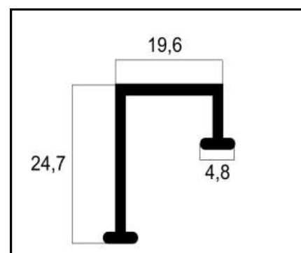
TC-11 DUPLO LIGHT / COMERCIAL PESO: 0,126 Kg/m
