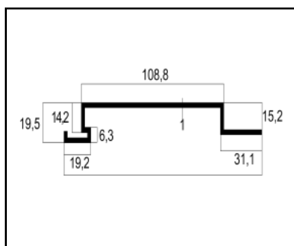
ALB-06 PESO: 0,643 Kg/m
