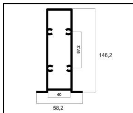
ALG-211 PERFIL COLUNA PESO: 1,917 Kg/m
