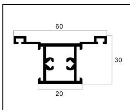
25-07 TRAVESSA PESO: 0,636 Kg/m
