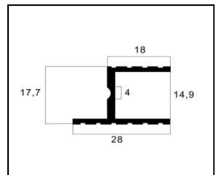
BXS-010 PESO: 0,270 Kg/m
