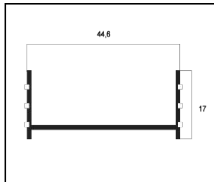
BXS-05 LATERAL PESO: 0,186 Kg/m
