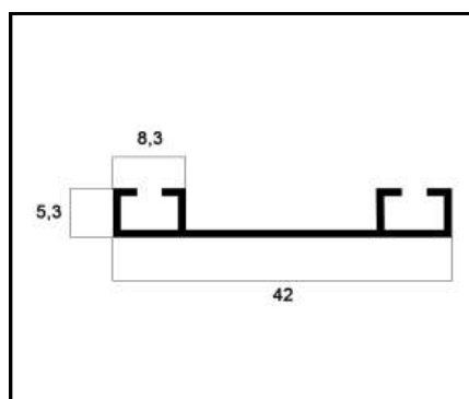
MV-098 TRILHO INFERIOR PESO: 0,135 Kg/m
