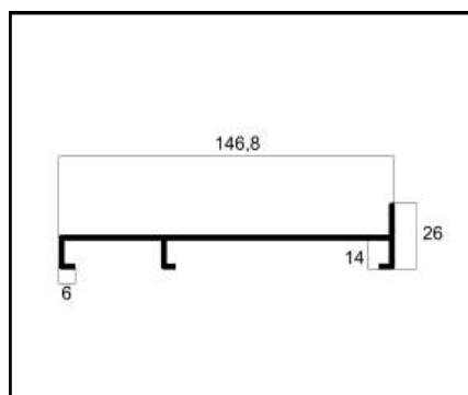
ALG-158 MARCO LATERAL 3 FOLHAS PESO: 0,865 Kg/m
