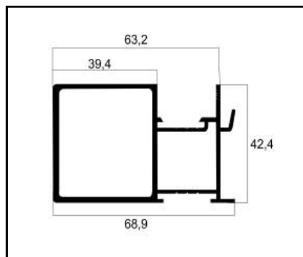
ASU-047 MÃO AMIGO INTERNO C/ REFORÇO PESO: 1,169 Kg/m
