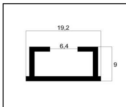
TS-04 TRILHO SUIÇO SEM ABA PESO: 0,099 Kg/m
