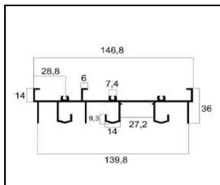
ALG-062 TRILHO SUPERIOR 3 FOLHAS PESO: 1,893 Kg/m
