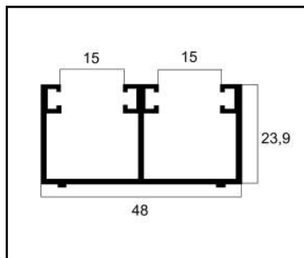
VT10-08 SUPERIOR DUPLO DESLIZANTE PESO: 0,559 Kg/m
