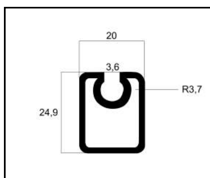
MV-02 PERFIL TRAVA DE TELA 25 X 20 PESO: 0,490 Kg/m
