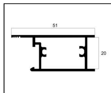
ASU-110 TRAVESSA PORTA DE GIRO PESO: 0,588 Kg/m
