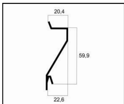
VZ-096 VENEZIANA LARGA CEGA PESO: 0,313 Kg/m
