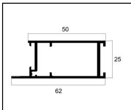
ASU-111 MONTANTE PORTA DE GIRO PESO: 0,702 Kg/m
