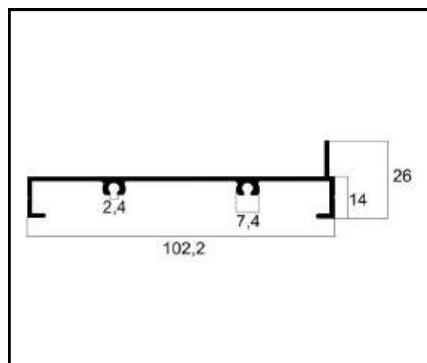
ALG-03 MONTANTE LATERAL 2 FOLHAS PESO: 0,806 Kg/m
