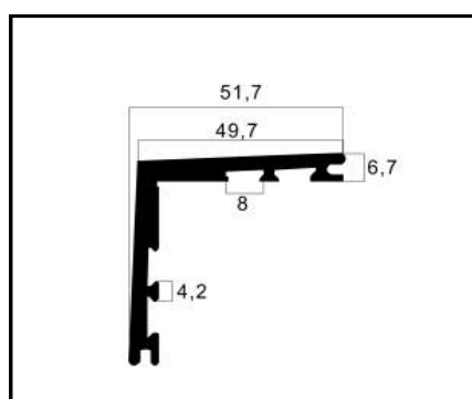
CL-09 (CL-06) CONEXÃO COM CUNHA PESO: 1,236 Kg/m
