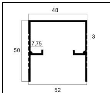
BXS-09 TRILHO SUPERIOR PESO: 0,508 Kg/m
