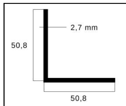
CL-036 CANTONEIRA 2 X 2,7MM PESO: 0,760 Kg/m
