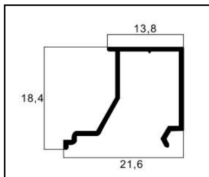
ASU-103 BAGUETE P/ MAXIM-AR PESO: 0,145 Kg/m
