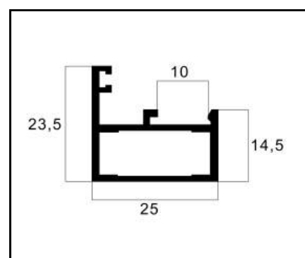
25-04 PESO: 0,334 Kg/m
