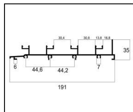
ALG-071 MARCO INFERIOR 4 FOLHAS PESO: 1,624 Kg/m
