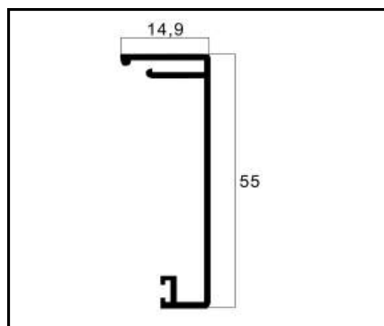
VT-09 CAPA PESO: 0,183 Kg/m
