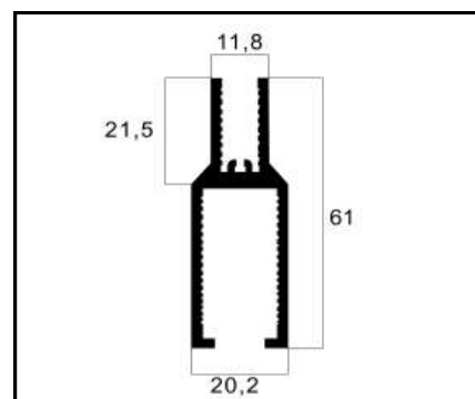
ALH-03 LEITO P/ VIDRO DESLIZANTE (SUPORTE) PESO: 0,764 Kg/m
