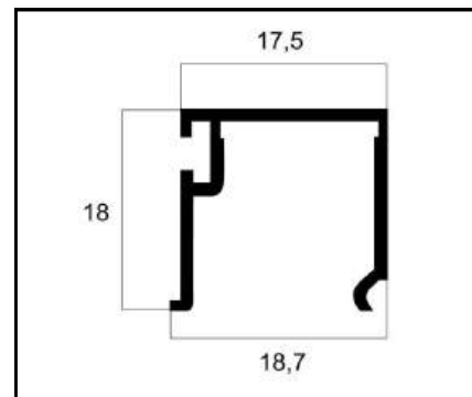
ALG-059 BATENTE LARGO PESO: 0,184 Kg/m
