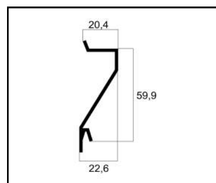
VZ-066 PALHETA PESO: 0,324 Kg/m
