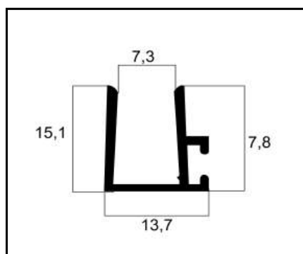
VT-128 TRANSPASSE PESO: 0,139 Kg/m
