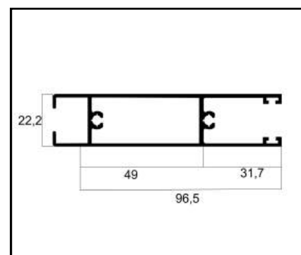
ASU-226 FOLHA INFERIOR HORIZONTAL PESO: 1,040 Kg/m
