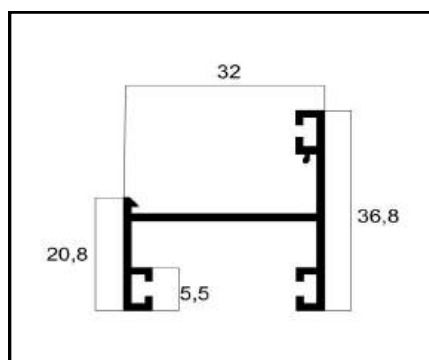
ALG-068 MARCO PESO: 0,418 Kg/m
