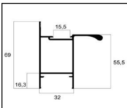
ALG-017 MONTANTE LAT C/ ABA PESO: 0,878 Kg/m
