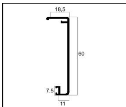
VT10-02 CAPA PESO: 0,299 Kg/m
