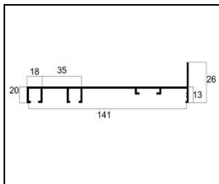
ASU-123 MARCO LATERAL CORRER 4 FOLHAS PESO: 0,838 Kg/m
