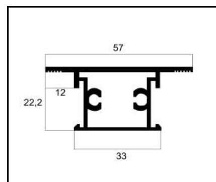
ASU-227 TRAVESSA CENTRAL DA FOLHA PESO: 0,493 Kg/m
