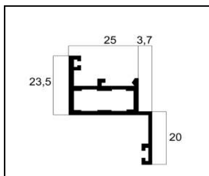
25-05 REQUADRO PESO: 0,500 Kg/m
