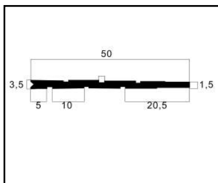
CL-08 (CL-011) CUNHA PESO: 0,356 Kg/m
