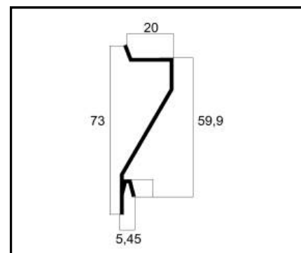
VZ-06 PALHETA LEVE PESO: 0,333 Kg/m
