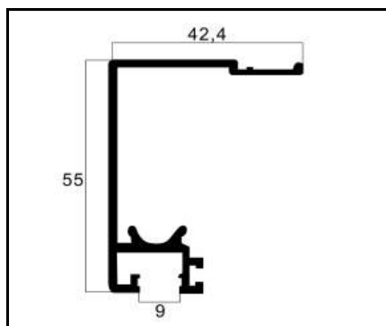
VT-08 TRILHO SUPERIOR PESO: 0,497 Kg/m
