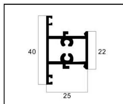
25-08 PESO: 0,541 Kg/m
