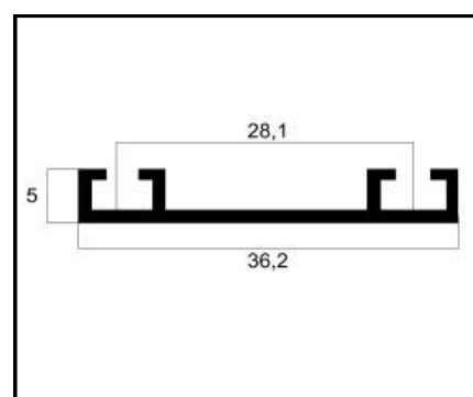
TI-063 TRILHO INFERIOR PESO: 0,114 Kg/m
