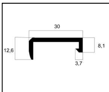
MV-01 PERFIL PARA ARCO DE MESA PESO: 0,315 Kg/m
