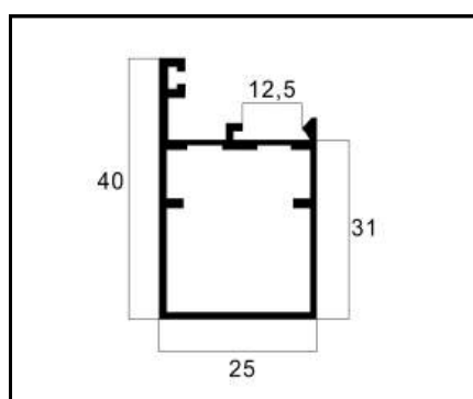
25-011 REQUADRO PESO: 0,490 Kg/m
