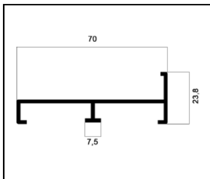
25-514 PESO: 0,521 Kg/m
