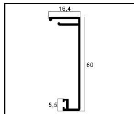
VT-225 CAPA PESO: 0,233 Kg/m
