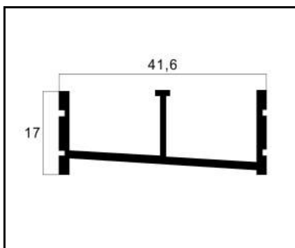
BXS-08 TRILHO INFERIOR E PESO: 0,230 Kg/m
