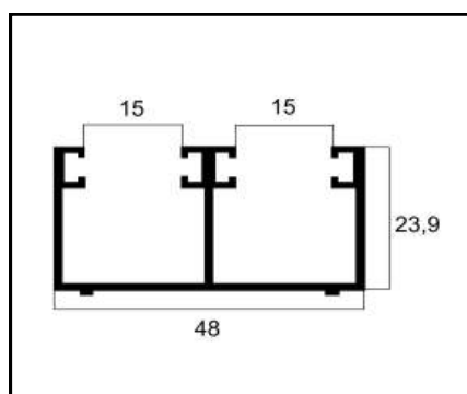
VT10-08 TRILHO INFERIOR DUPLO P/ STANLEY PESO: 0,559 Kg/m
