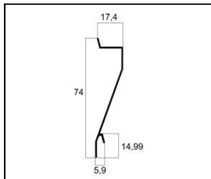
VZ-03 VENEZIANA MEDIA CEGA PESO: 0,255 Kg/m
