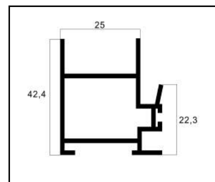
ASU-556 MONTANTE MÃO DE AMIGO PESO: 0,577 Kg/m
