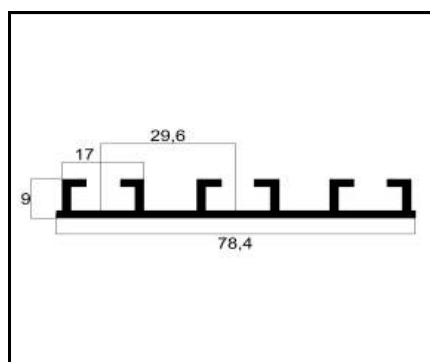
TS-03 TRILHO SUIÇO TRIPLO MAX PESO: 0,345 Kg/m
