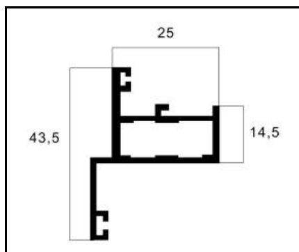
25-205 REQUADRO PESO: 0,454 Kg/m
