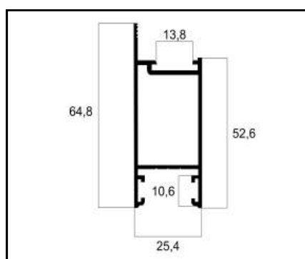
ASU-245 FOLHA LATERAL VERTICAL PESO: 0,607 Kg/m
