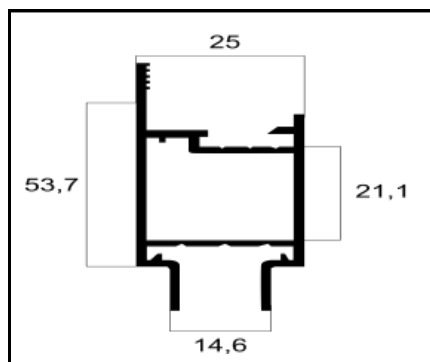
ASU-192 FOLHA CENTRAL VERTICAL PESO: 0,435 Kg/m
