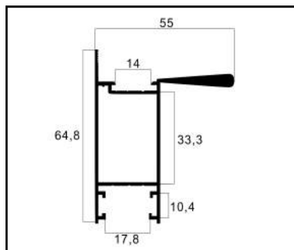
ASU-280 ALTURA DA FOLHA C/ PUXADOR PESO: 0,895 Kg/m
