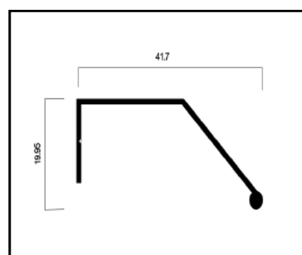
MV-069 PUXADOR PESO: 0,253 Kg/m
