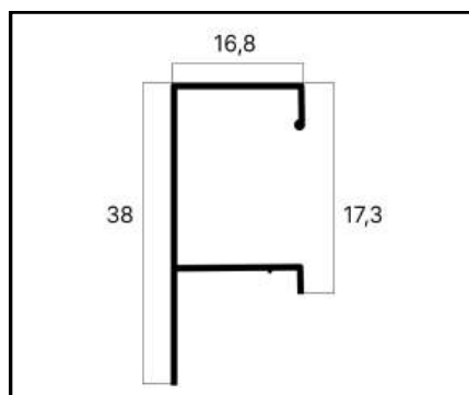
MV-095 PUXADOR LEVE PESO: 0,210 Kg/m
