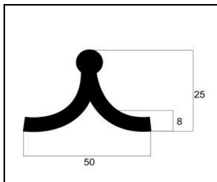
DS-136 PERFIL QUILHA PESO: 0,869 Kg/m
