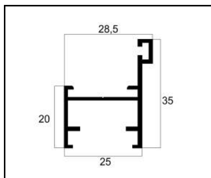
ASU-079 MARCO PESO: 0,359 Kg/m
