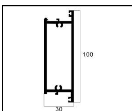
30-030 PESO: 1,224 Kg/m
