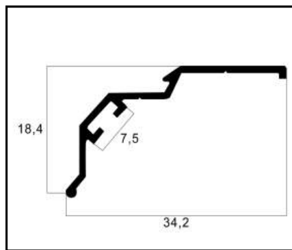
ASU-083 PINGADEIRA PESO: 0,141 Kg/m
