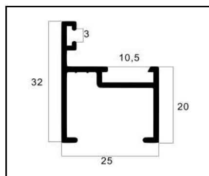
25-311 PESO: 0,330 Kg/m
