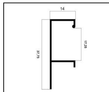
MV-097 PUXADOR PESO: 0,130 Kg/m
