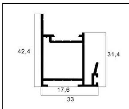
ASU-041 MÃO DE AMIGO EXTERNO PESO: 0,475 Kg/m
