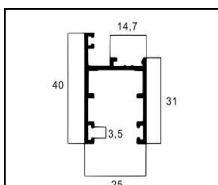
25-014 REQUADRO L-25 PESO: 0,434 Kg/m
