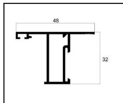
ALG-085 TRAVESSA PESO: 0,575 Kg/m
