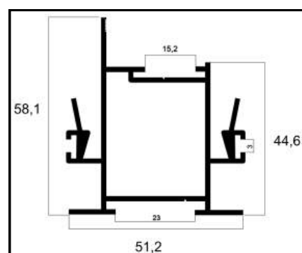
ALG-162 MONTANTE MÃO AMIGO PESO: 1,041 Kg/m
