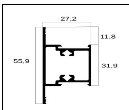
30-017 TRAVESSA PESO: 0,658 Kg/m
