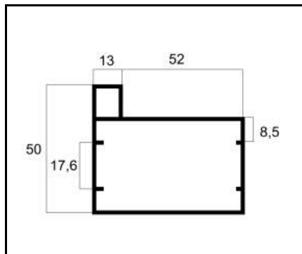
AMT-01 MONTANTE 65 PESO: 0,674 Kg/m
