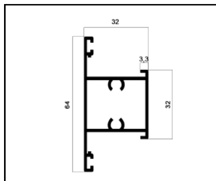
ALG-074 PERFIL COLUMNA PESO: 0,691
