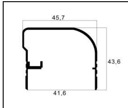
BXS-02 CHAPÉU REDONDO PESO: 0,505 Kg/m
