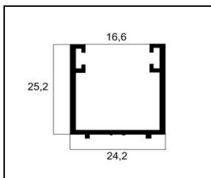
VT-054 SUPERIOR SIMPLES DESLIZANTE PESO: 0,282 Kg/m
