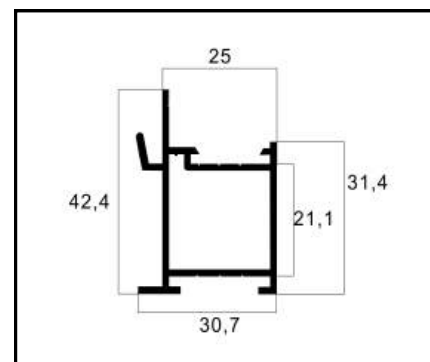
ASU-040 MÃO DE AMIGO INTERNO PESO: 0,451 Kg/m
