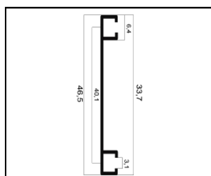
MV-093 TRILHO INFERIOR PESO: 0,152 Kg/m
