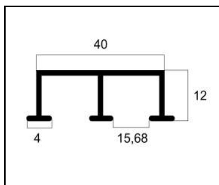
TC-12 TRILHO LIGHT PESO: 0,148 Kg/m
