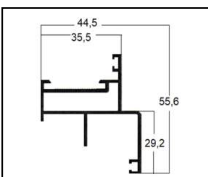
30-027 PESO: 0,782 Kg/m
