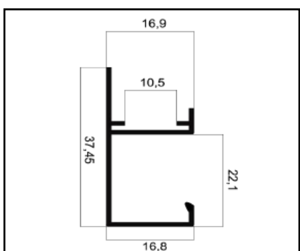
MV-091 PUXADOR PESO: 0,163 Kg/m
