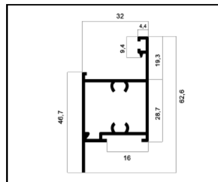
ALG-076 TRAVESSA PESO: 0,597
