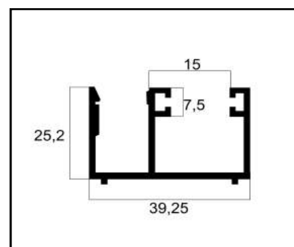
VT10-03 TRILHO INFERIOR PESO: 0,394 Kg/m
