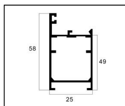
25-023 REQUADRO PESO: 0,662 Kg/m
