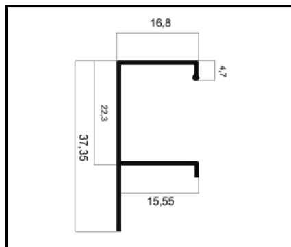
MV-096 PUXADOR PESO: 0,130 Kg/m
